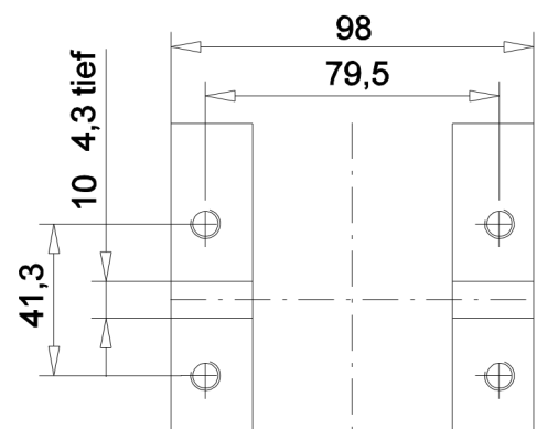
Maße - Getriebefuß
